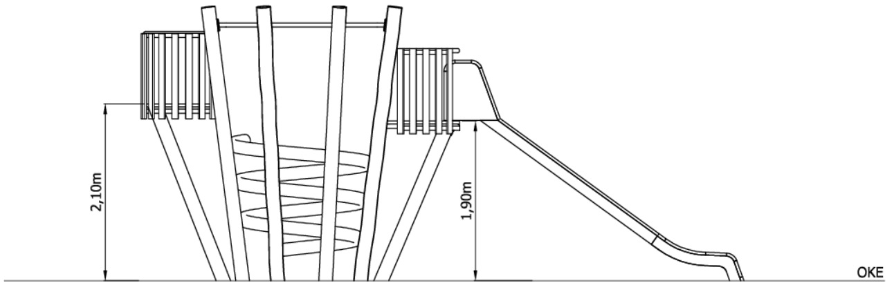
Ansicht M -1:50-
