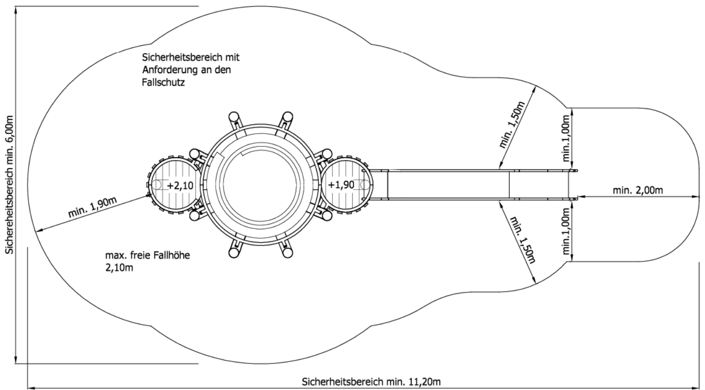
Draufsicht M-1:50-
